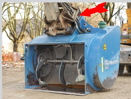
Flüssigbodenschaufel + Verbauzieher
